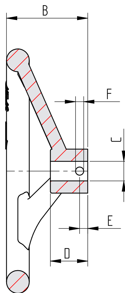
Doorsnede B-B
